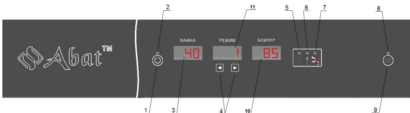
Рис. 1. Устройство посудомоечной машины
