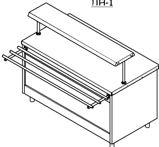
ПН-1
