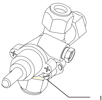
Рис. 5: Газовый кран
